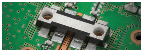
V/UHF帯 ファイナルMOS FET RD70HUF2
