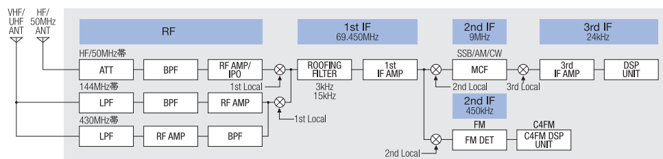
受信ブロックダイアグラム
